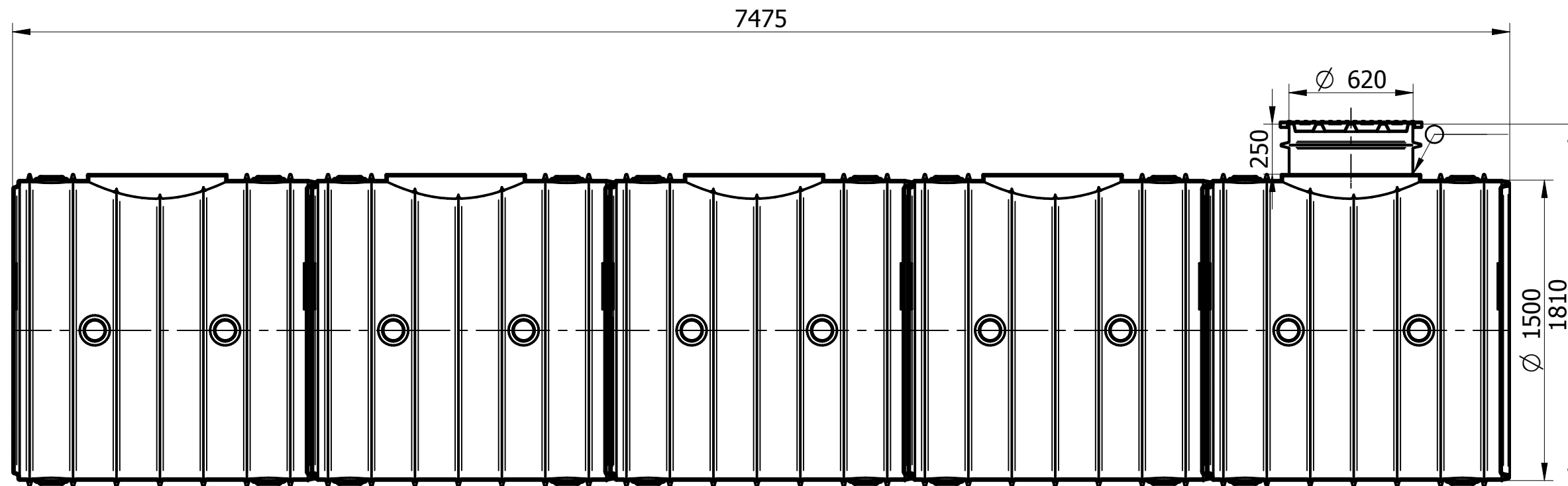
METSZET A-A
